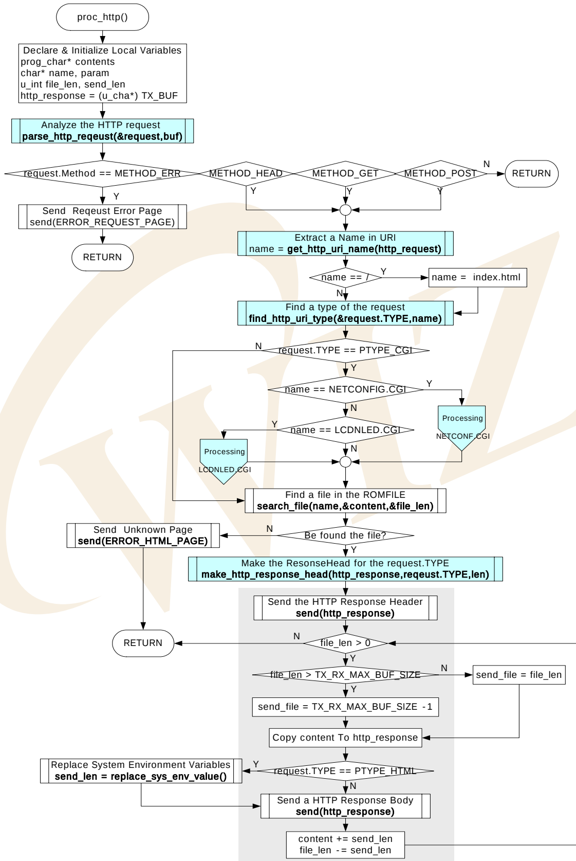
<Fig 3.19: proc_http()>
