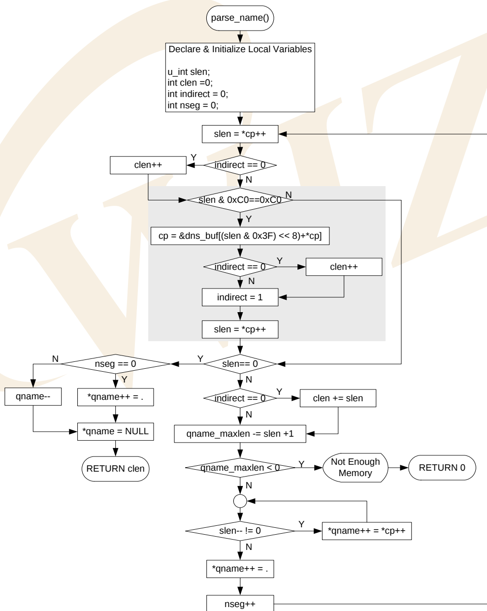
<Fig 3.44: parse_name()>
