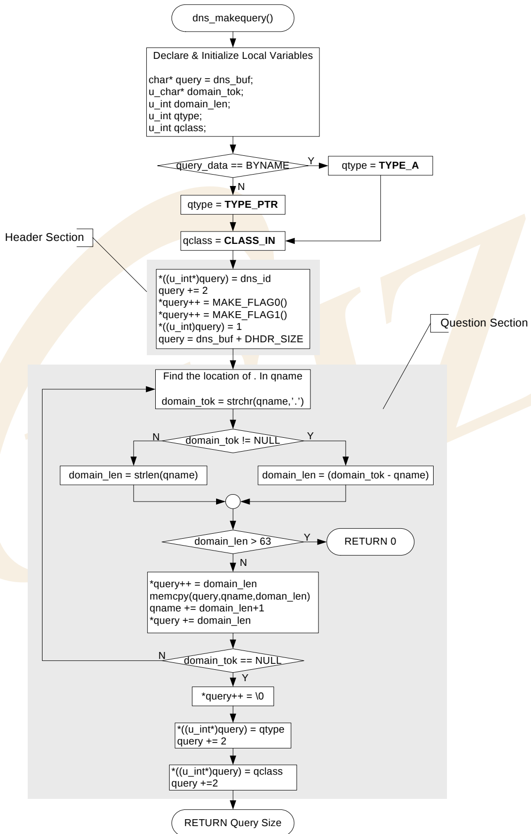
<Fig 3.40: dns_makequery()>
