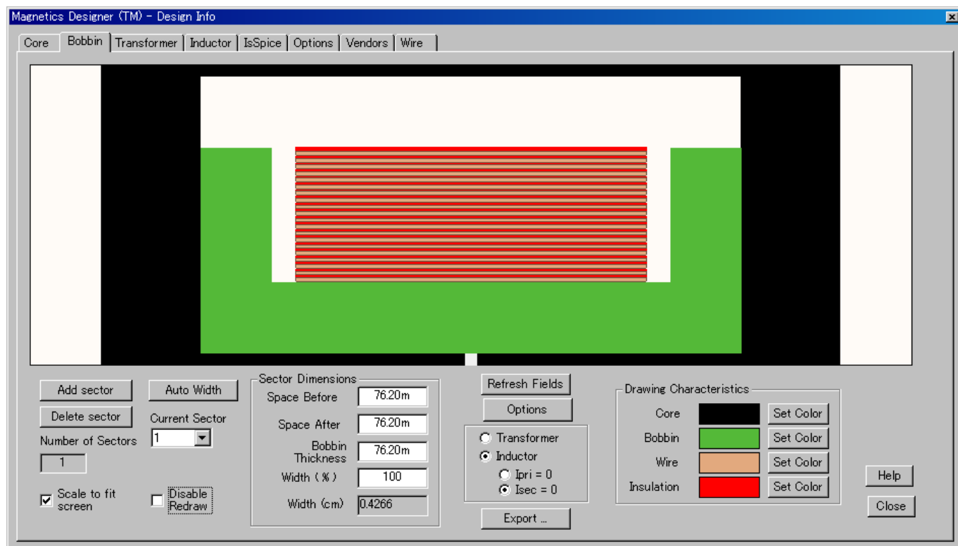
図 3. Foil テーブル使用例( 銅箔 )
