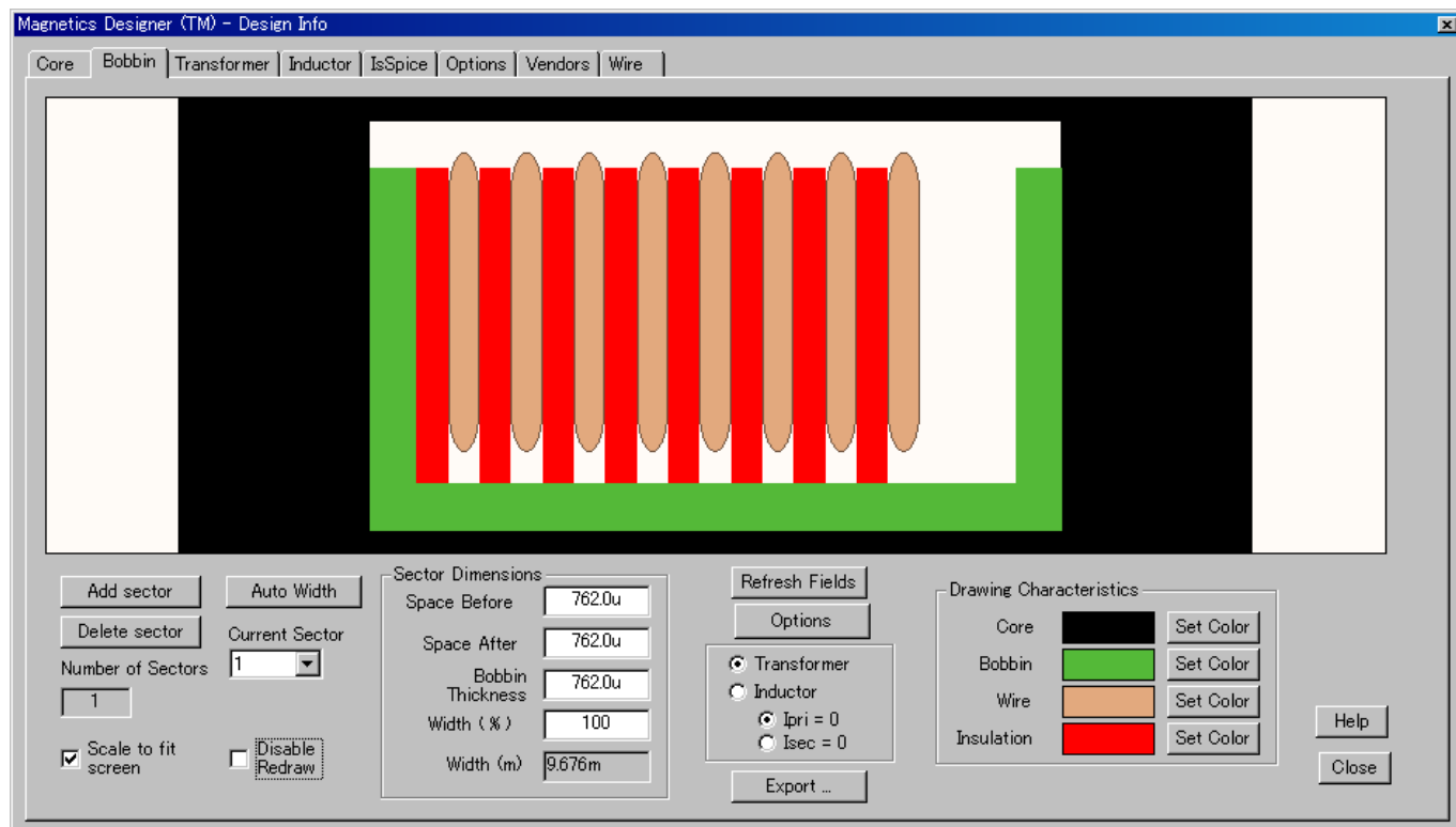
図 4. PCB テーブル使用例( プリントコイル )
