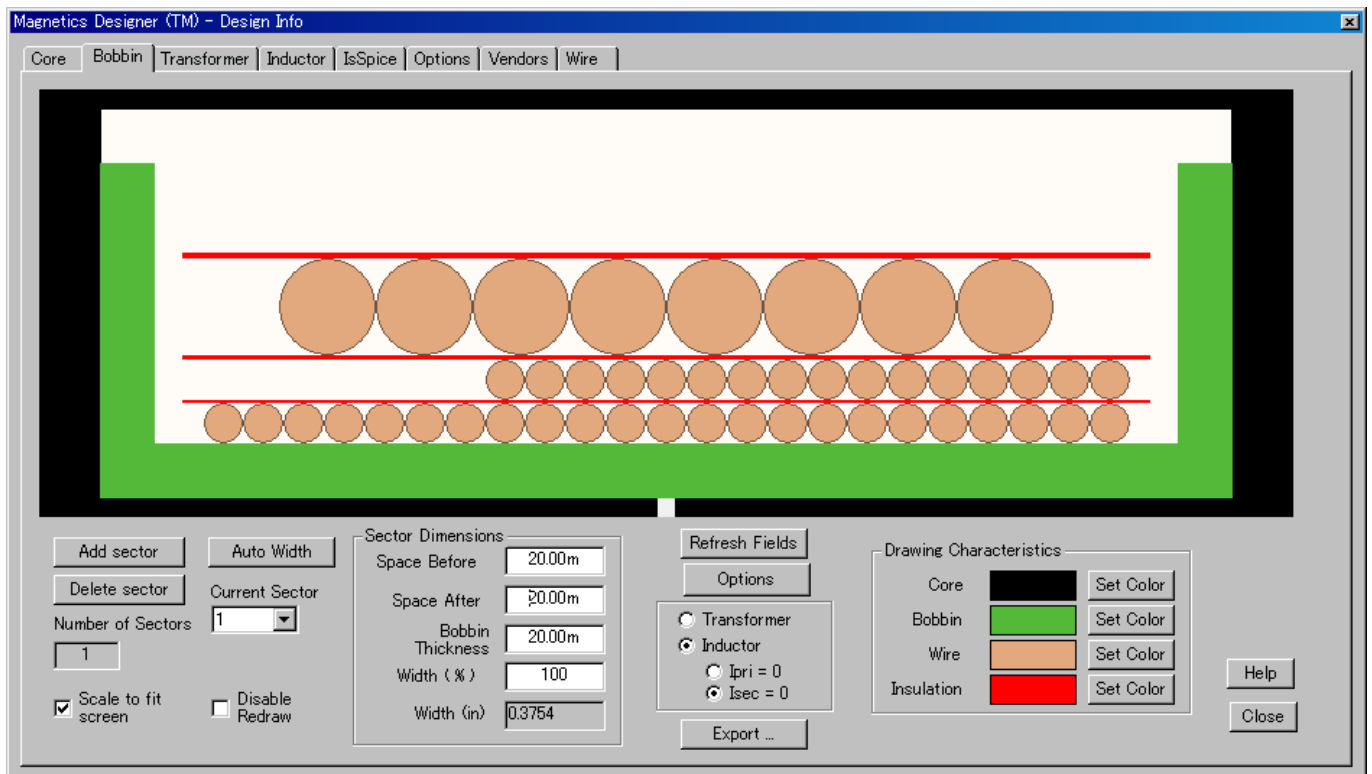
図 1. 円形ワイヤ使用例
