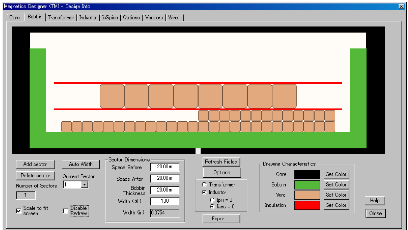
図 2. 四角形ワイヤ使用例
